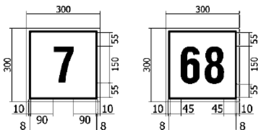
Глубина светового короба 80-130 мм.
